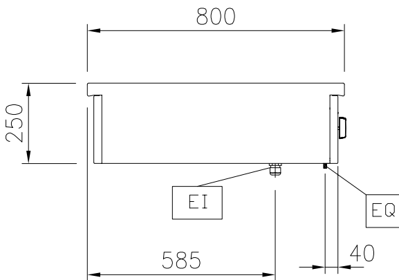
Zij aanzicht
